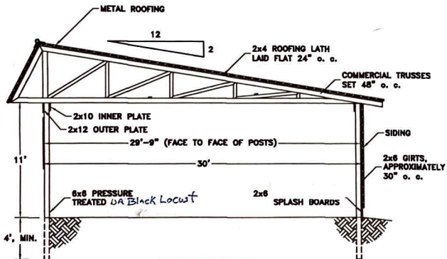
CROSS SECTION SCALE: 1/8" = 1'-0"
